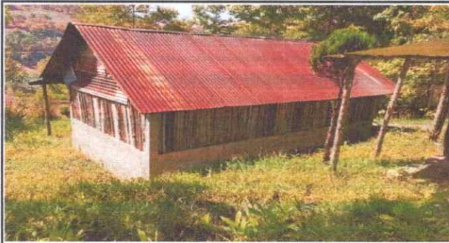
Foto 1: Vista panorámica del centro estudiantil, cuenta con cuatro hiladas de block, que es necesaria la sustitución de parales
